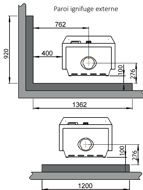
Paroi ignifuge externe
