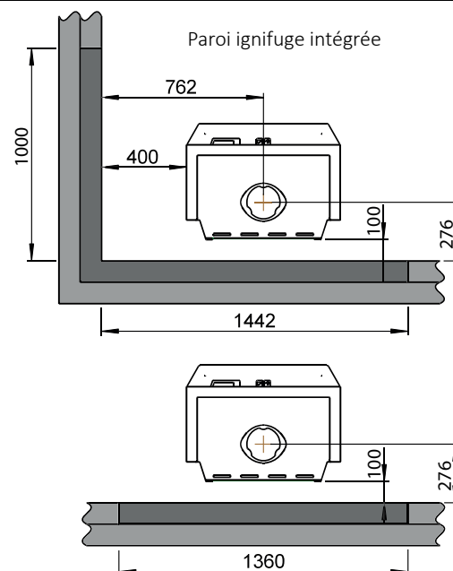
Paroi ignifuge intégrée
